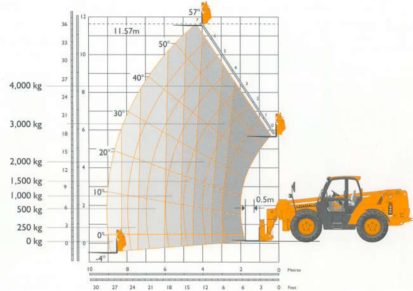
Nivelación de Chasis (Sway) Con estabilizadores recogidos (Angulo de nivelación ± 9°)
