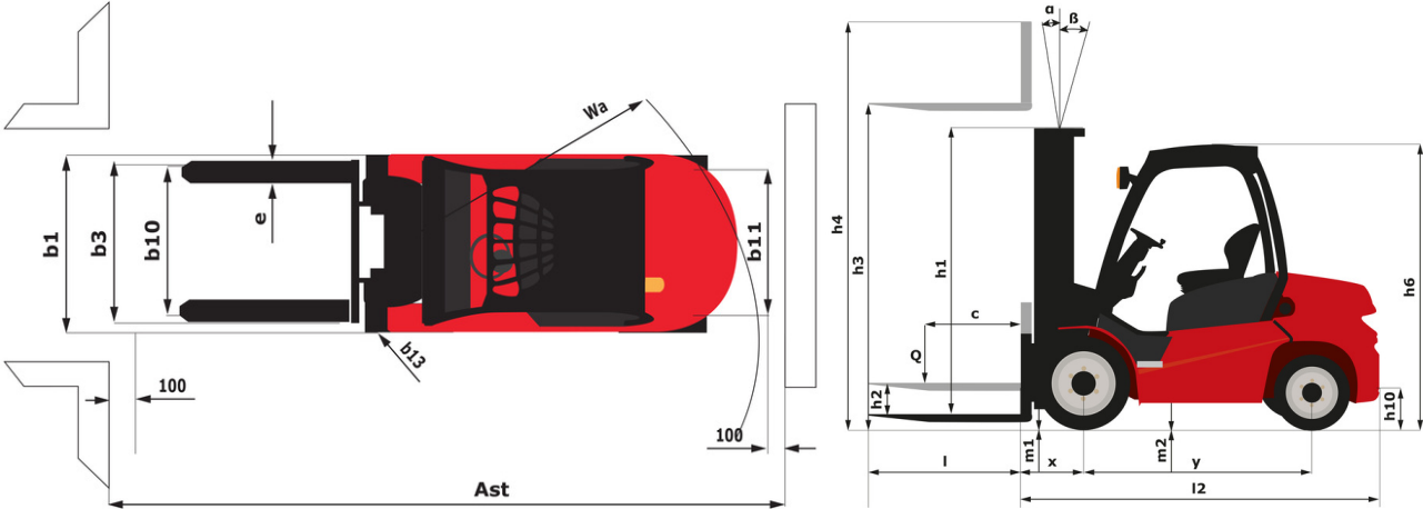
MI 25 D ST5 - Diagrama dimensional
